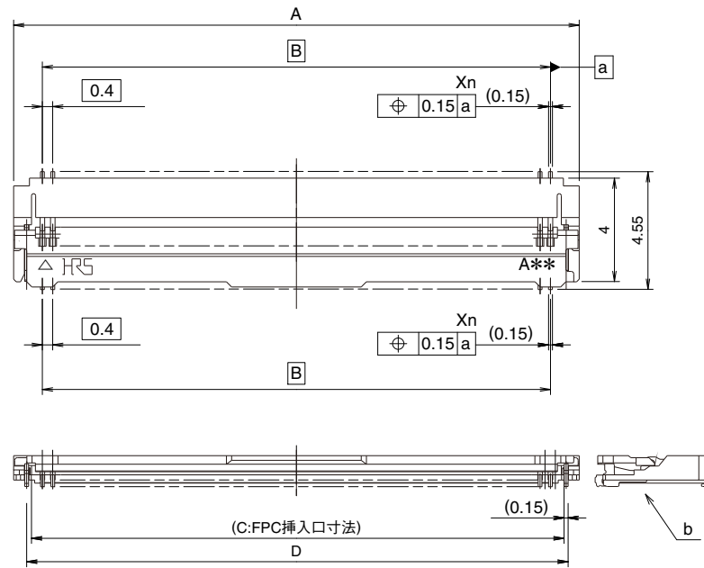
b 詳細図
