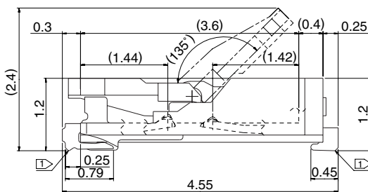
b 詳細図
