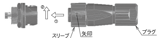
ロック構造図
