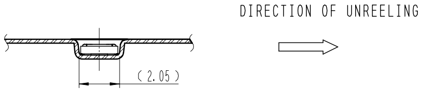
C-C (5:1)
