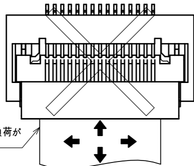
補強フィルム(斜め)
