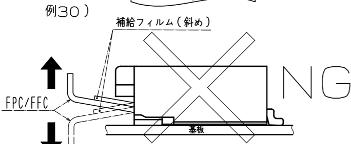
FPC/FFCに負荷が掛かった状態
