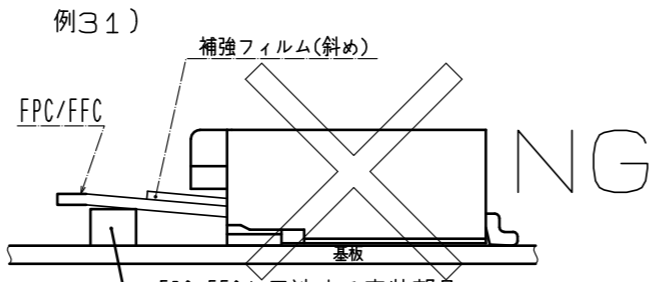
FPC/FFCと干渉する実装部品
