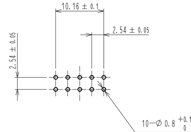
推奨基板寸法図
