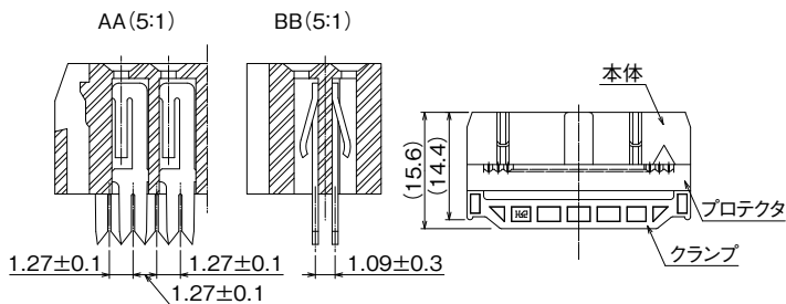
■A-A断面図
