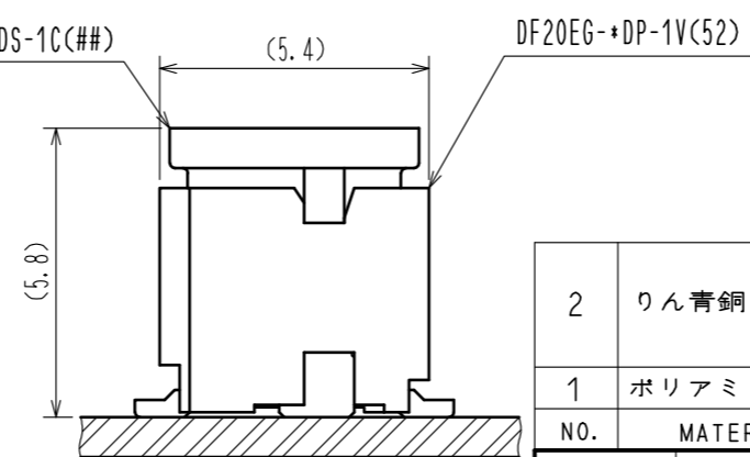
ソケット嵌合図
