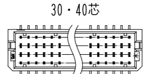
2 リブの本数及び位置
