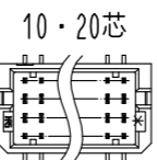
2 リブの本数及び位置
