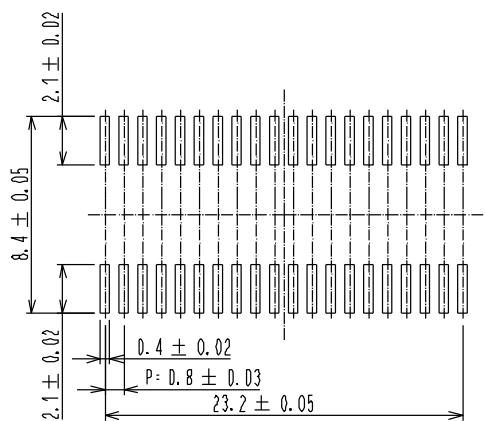
信号部パターン(C 部)詳細
