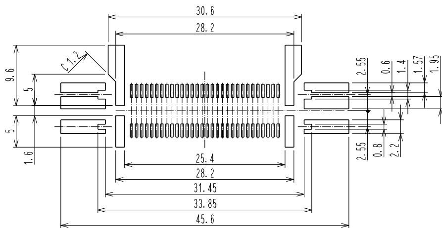
MF 端子部パターン(D 部)詳細
