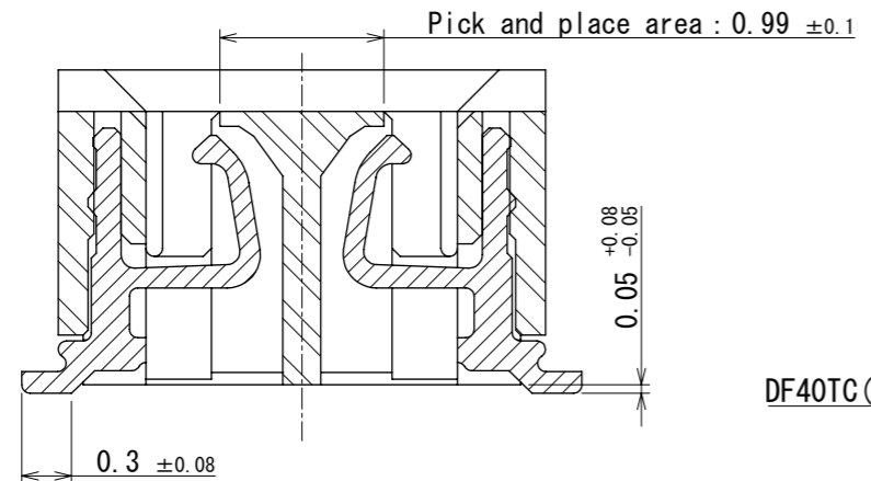
A-A (20 : 1)
