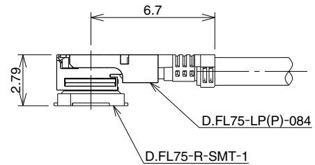
嵌合外観図
