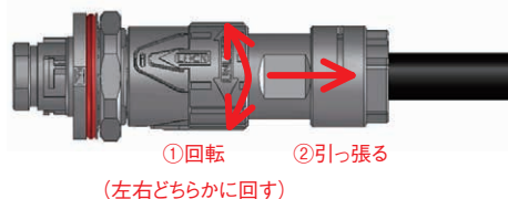
ロック構造(プッシュオン・バヨネット)
