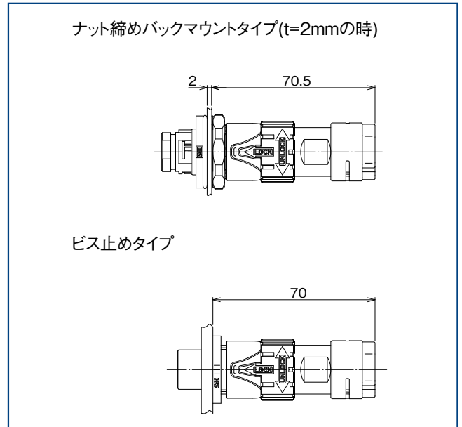
嵌合状態図
