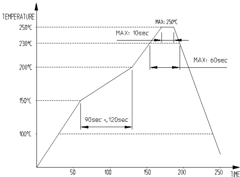
[Fig1]. 推奨リフロープロファイル
