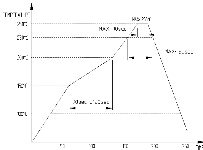
図-1 リフロープロファイル
