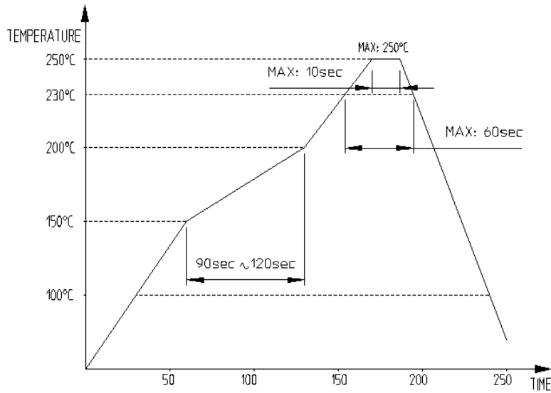
図-1 リフロープロファイル
