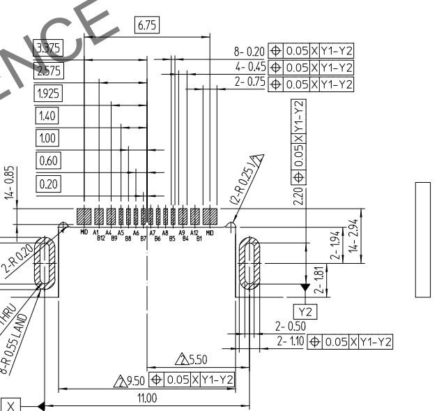
△ RECOMMENDED PCB LAYOUT (TOP-VIEW) (推奨PCBレイアウト上面図) (GENERAL TOLERANCE : ±0.05) (一般的な許容範囲)
