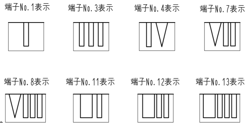
1 図-1 端子No.表示(10:1)
