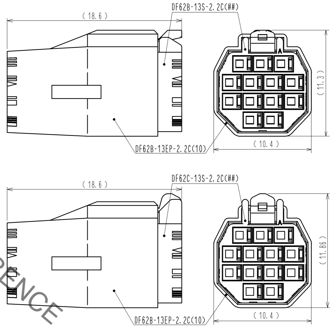
嵌合状態図(FREE)
