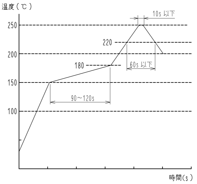
鉛フリークリームはんだ温度プロファイル (推奨)
