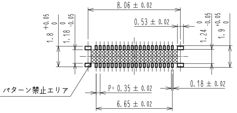
△◆推奨パターン図
