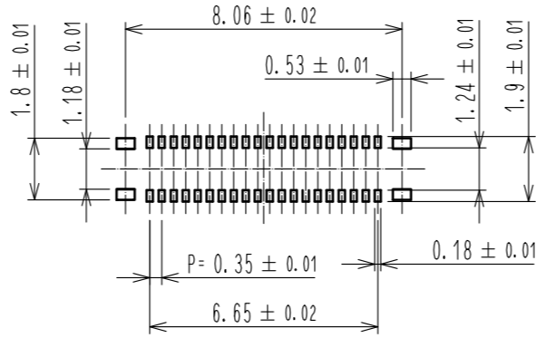
△◆メタルマスク開口部推奨加工図 メタルマスク厚さ: 80μm
