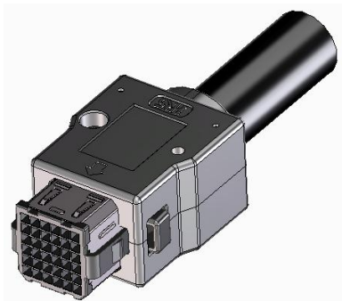
コネクタ各部名称
