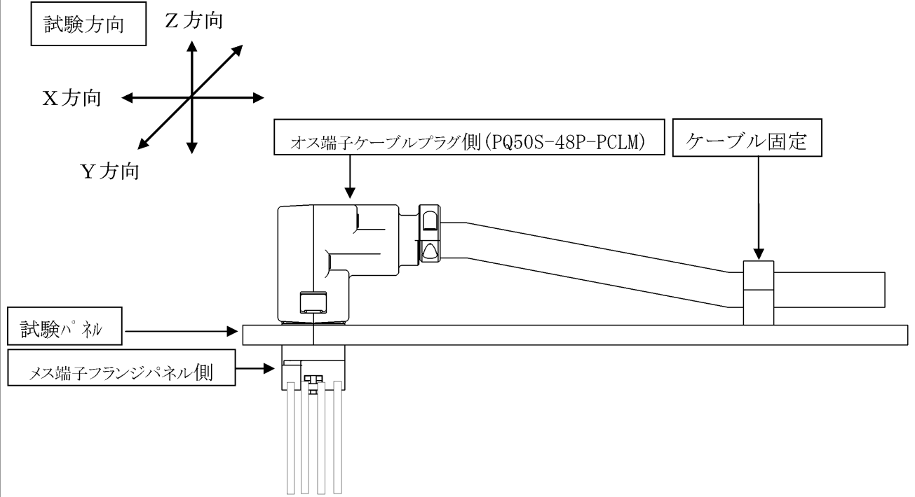
オス端子ケーブルプラグ&メス端子フランジパネル振動試験方法概略図 (側面)
