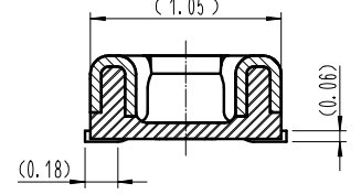
B-B (30:1)
