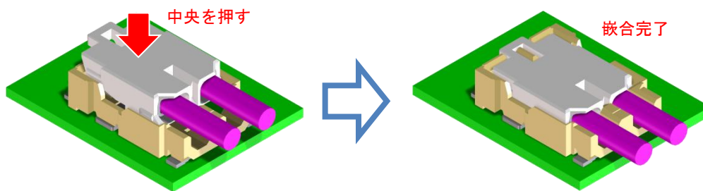
図 3. 挿入作業
