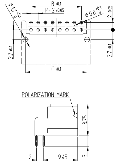
Unit : mm
