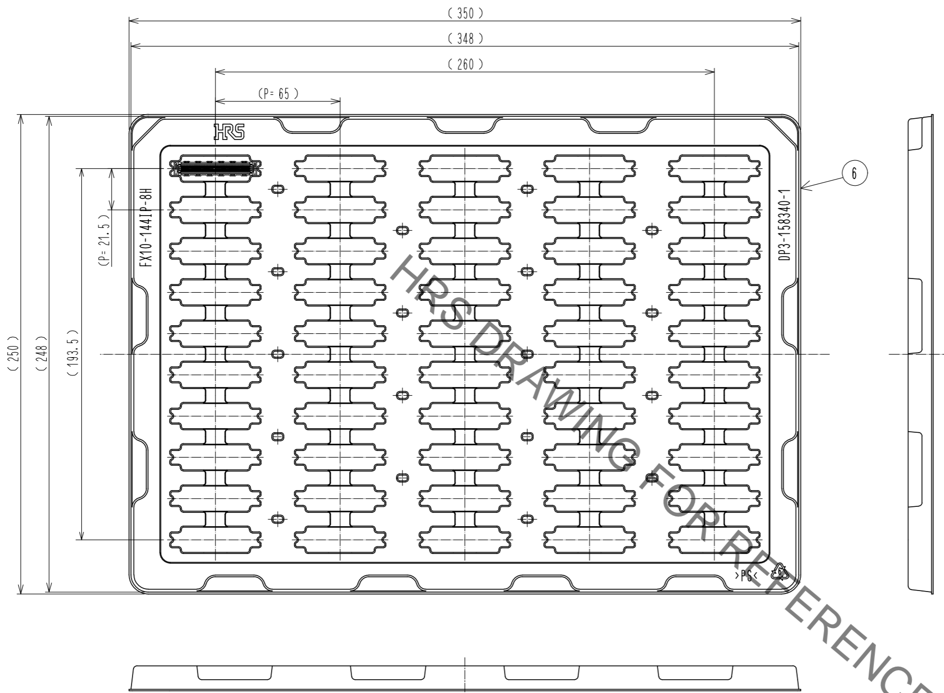
Fig. 3 梱包状態図 (1:2) ◁ 6
