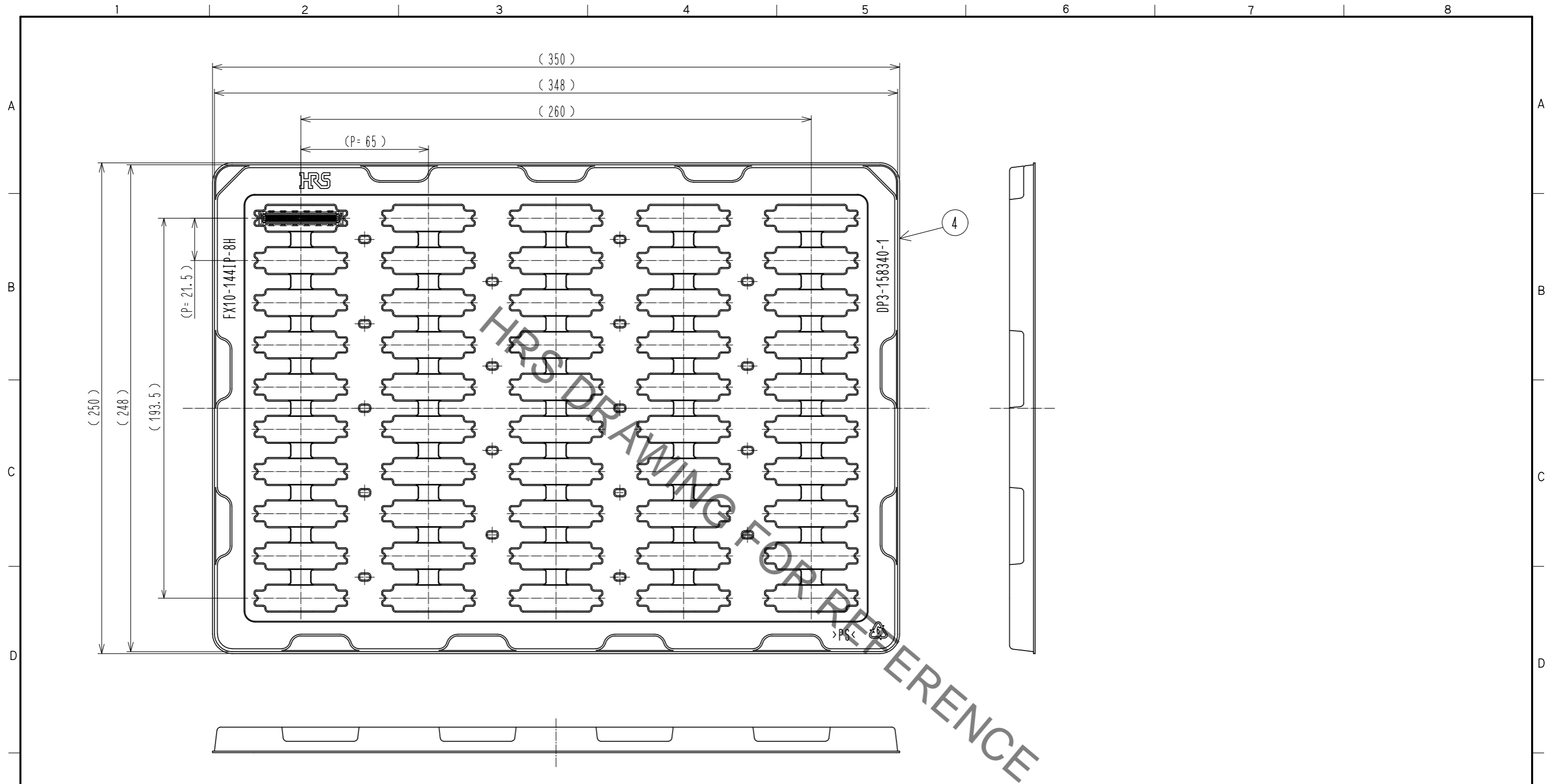
Fig.3 梱包状態図 (1:2) ◁6
