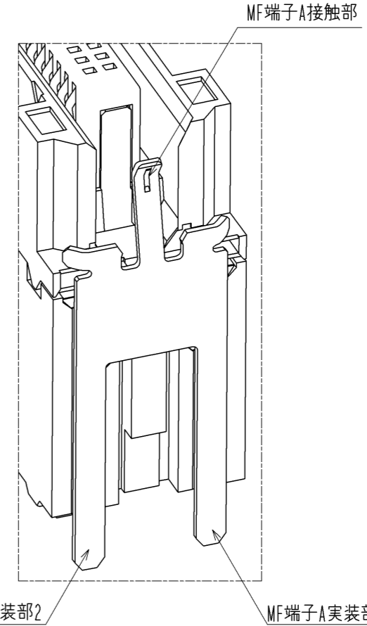
⑧ MF端子A構造
