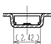
C-C (5:1)
