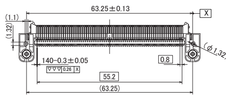
ER8L-140P-0.8SH(##)
