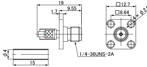
HRM-200-3S-1C
