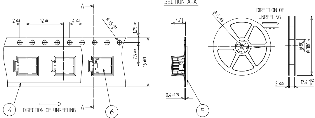
SECTION A-A
