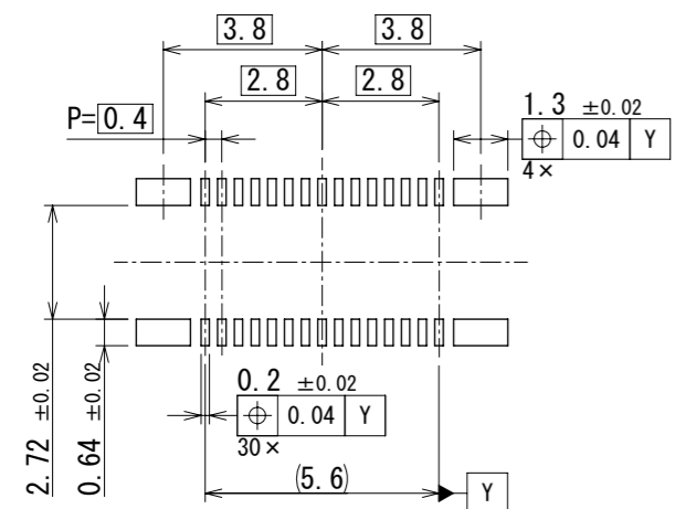
推奨基板レイアウト (5:1) △
