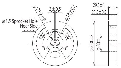
Reel Dimensions
