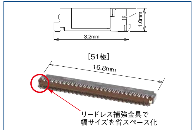
高さ1.0mm、実装奥行き3.2mmを実現
