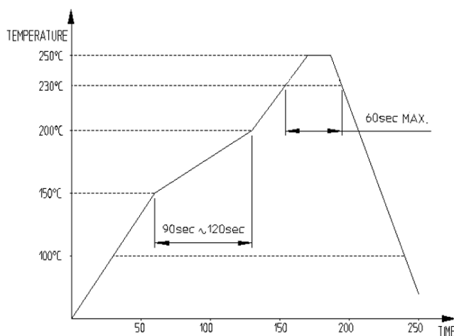
[図-1]. 推奨リフロースタットプロファイル
