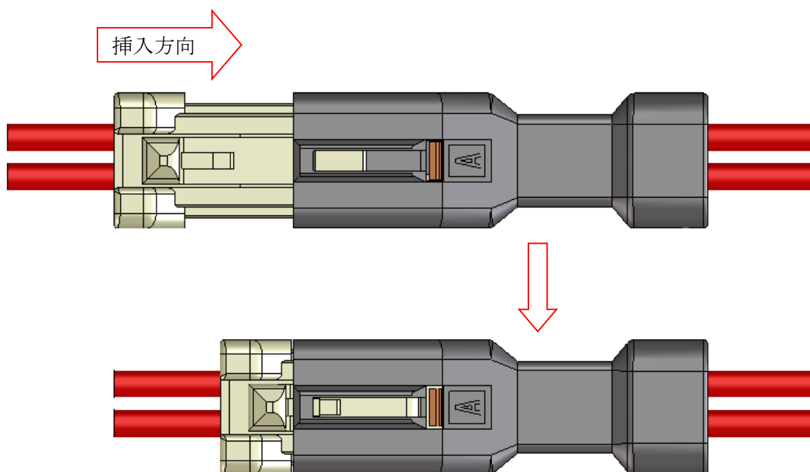
図 4. 挿入方法
