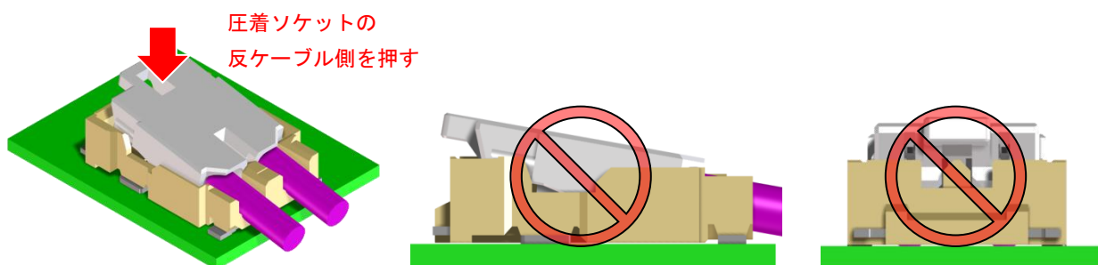
図 5. 未嵌合嵌合状態
