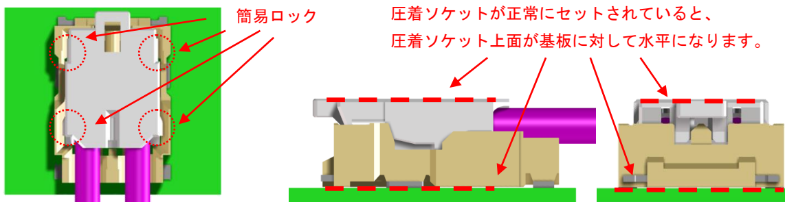
図 2. 圧着ソケットのセット方法
