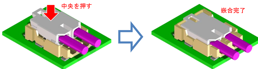
図 3. 挿入作業
