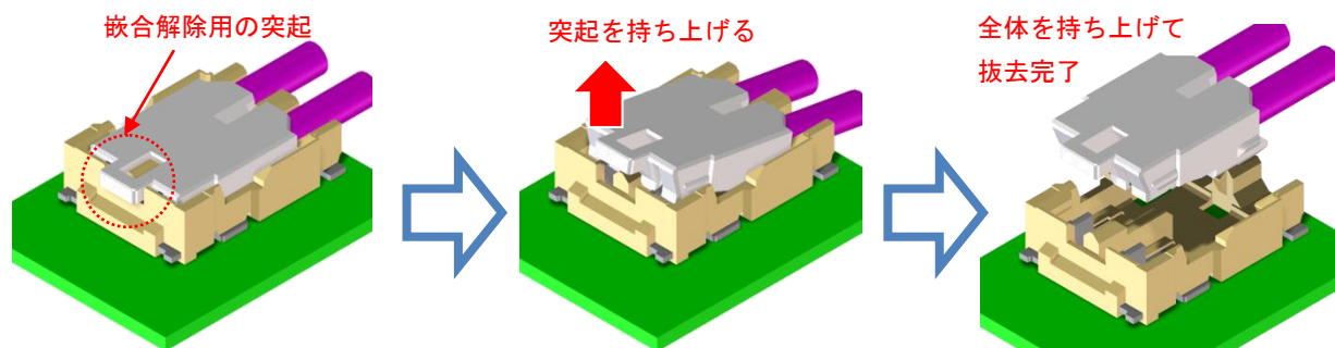
図 7. 抜去方法
