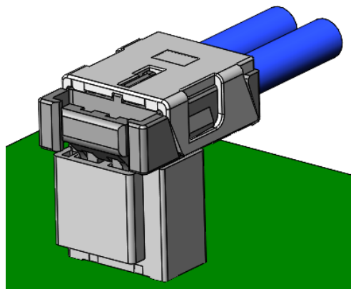
図 7. 嵌合状態
